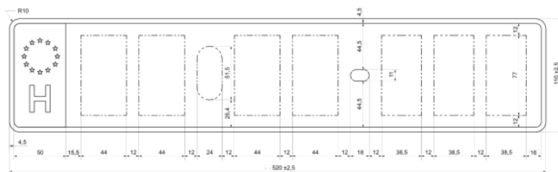
1. ábra: „A” és „D” típusú rendszámtáblák rajzai
